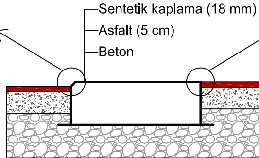
A-A KESİTİ
